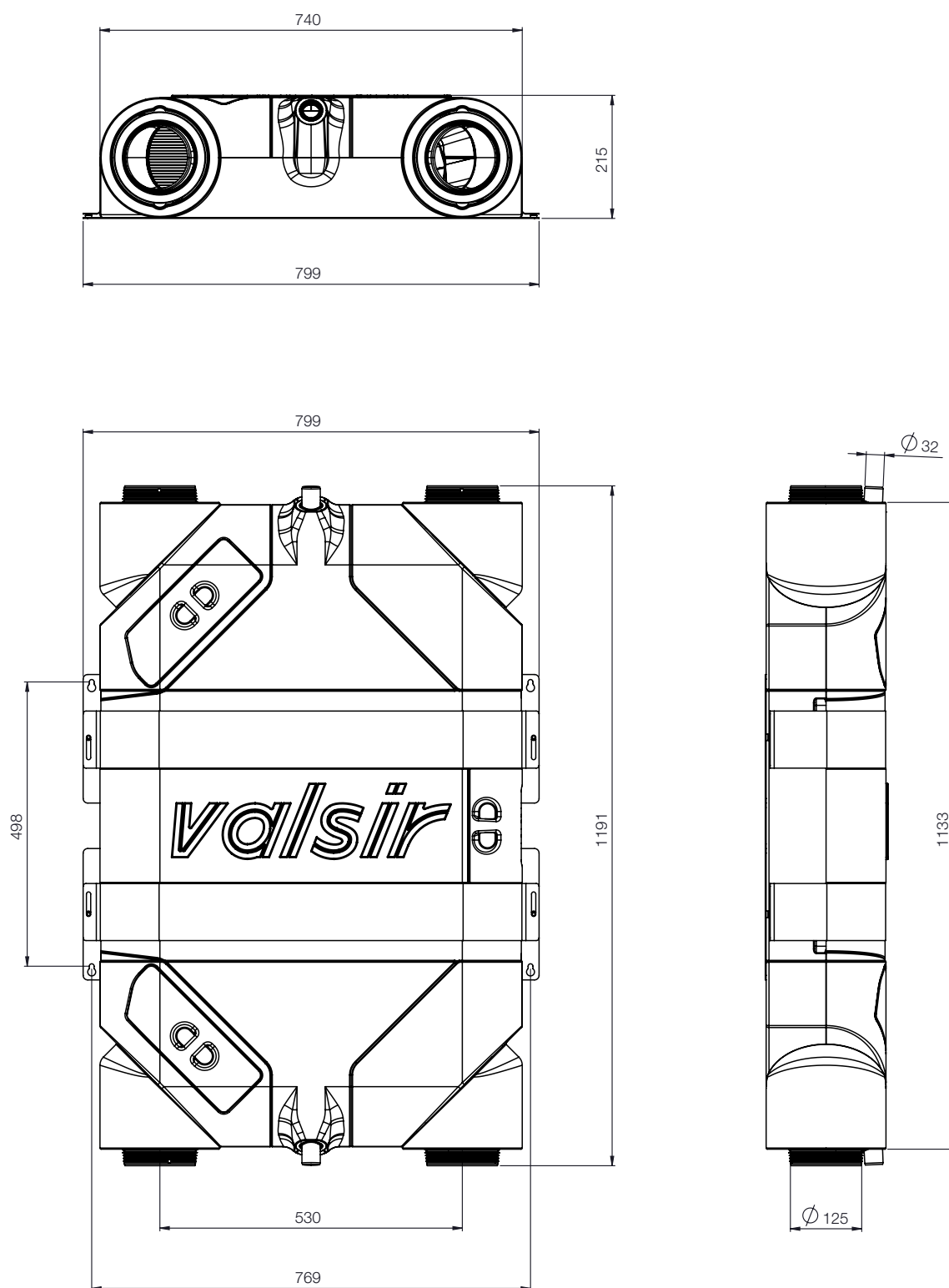
Obrázek 1 Kótovaný výkres jednotky Ariosa HV.
