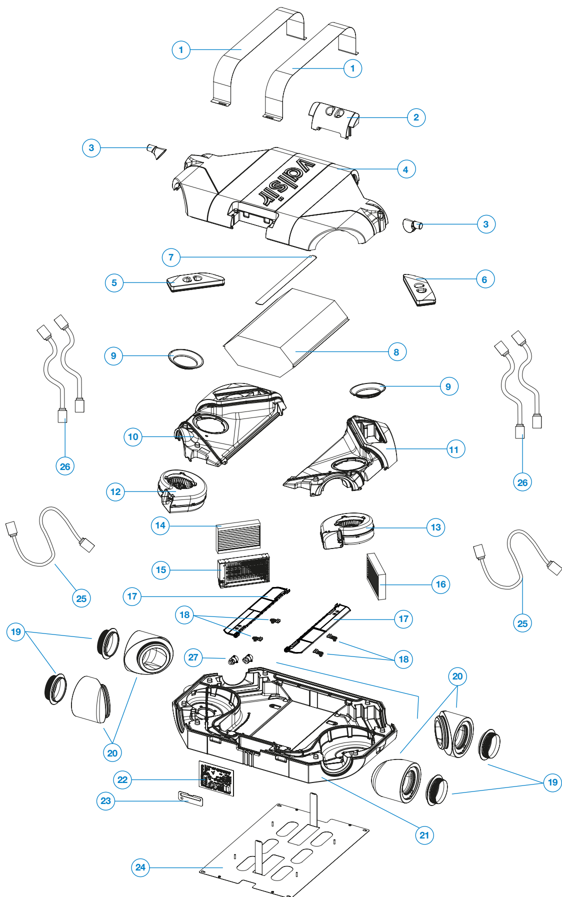
Obrázek 4 Součásti jednotky Ariosia HV.
